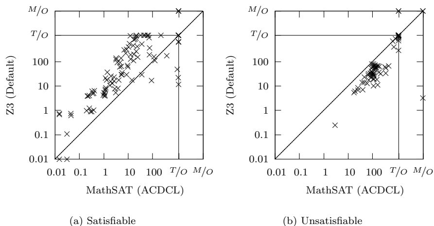
Fig. 6: MathSAT (ACDCL) vs Z3 Default.
